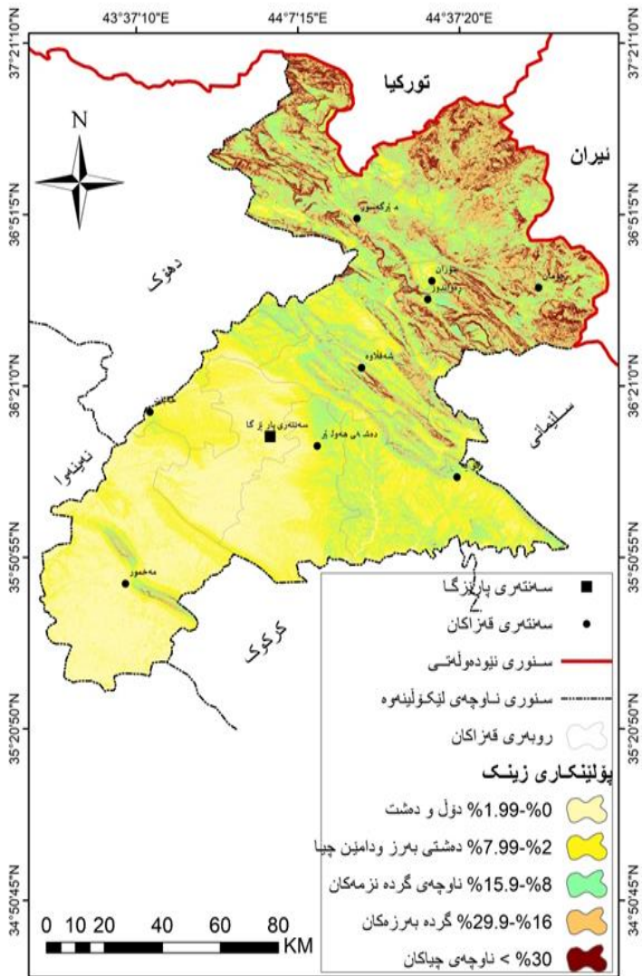
سەرچاوە: تۆپۆر بەبەکارھێنانى (DEM) ى 30 مەترى لەرێگەى پرۆگرامى (ArcGis10.8)
