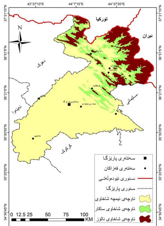
سه رجاوه: توێژه به بهكارهینانی (DEM) ی 30 مهتری له رنگی پرۆگرامی (ArcGis10.8)
