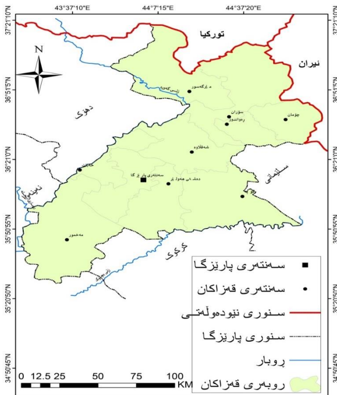
سەرچاوه: توێژه‌ر به‌به‌کارهینانی (DEM) ی 30 مه‌تری له‌ریگه‌ی پرۆگرامی (ArcGis10.8)
